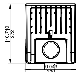
EEL-AL50W Dimensions mm | 272(L) x 230(W) x 69(H) inch | 10.7(L) x 9(W) x 2.7(H)
