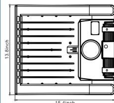
EEL-AL150W Dimensions mm | 391(L) x 350(W) x 71(H) inch | 15.4(L) x 13.8(W) x 2.8(H)
